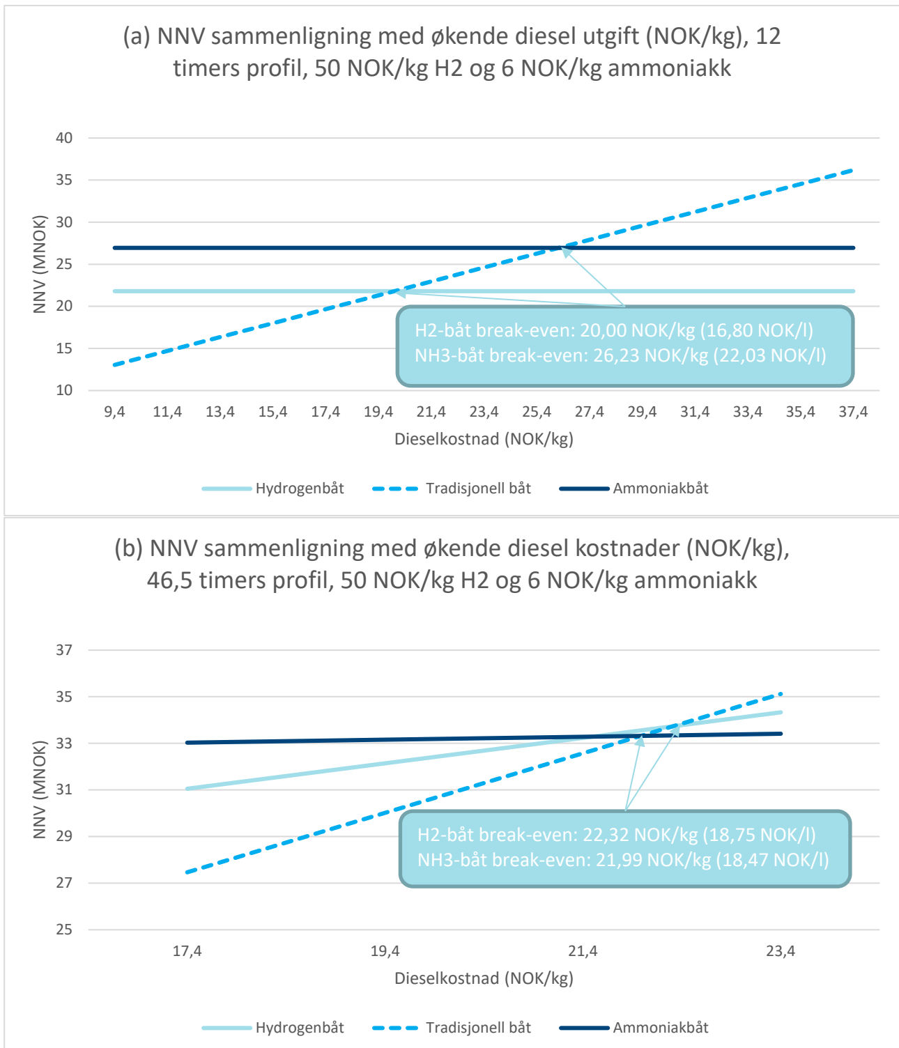
Figur 5-19 Nettonåverdi (NNV) sammenligning mellom de ulike kostnader med økende dieselskostnader for casene med 50 kr/kg H 2 og 6 kr/kg NH 3 (ammoniakk) for de to profilene, i den øverste grafikken (a) ser man resultater på en 12 timers profil, mens på den nederste (b), er det for en 46,5 timers profil
